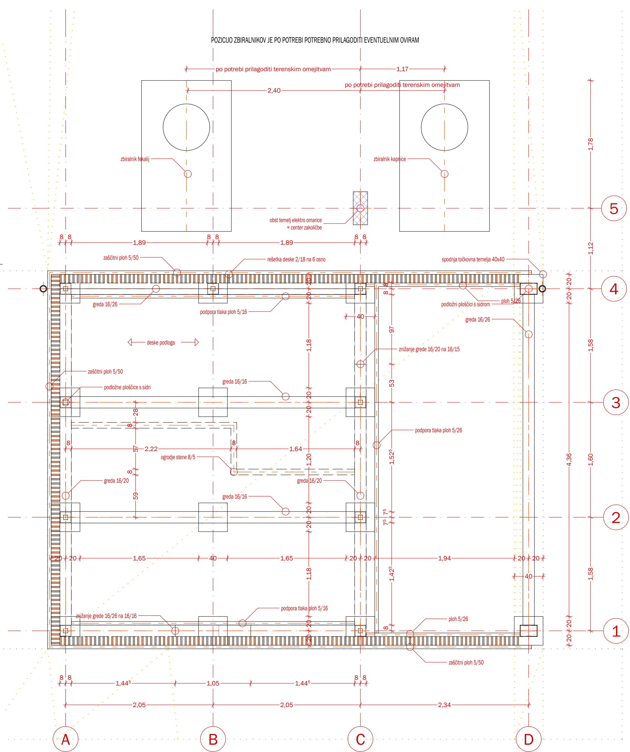
1. temelji novo 1:25
