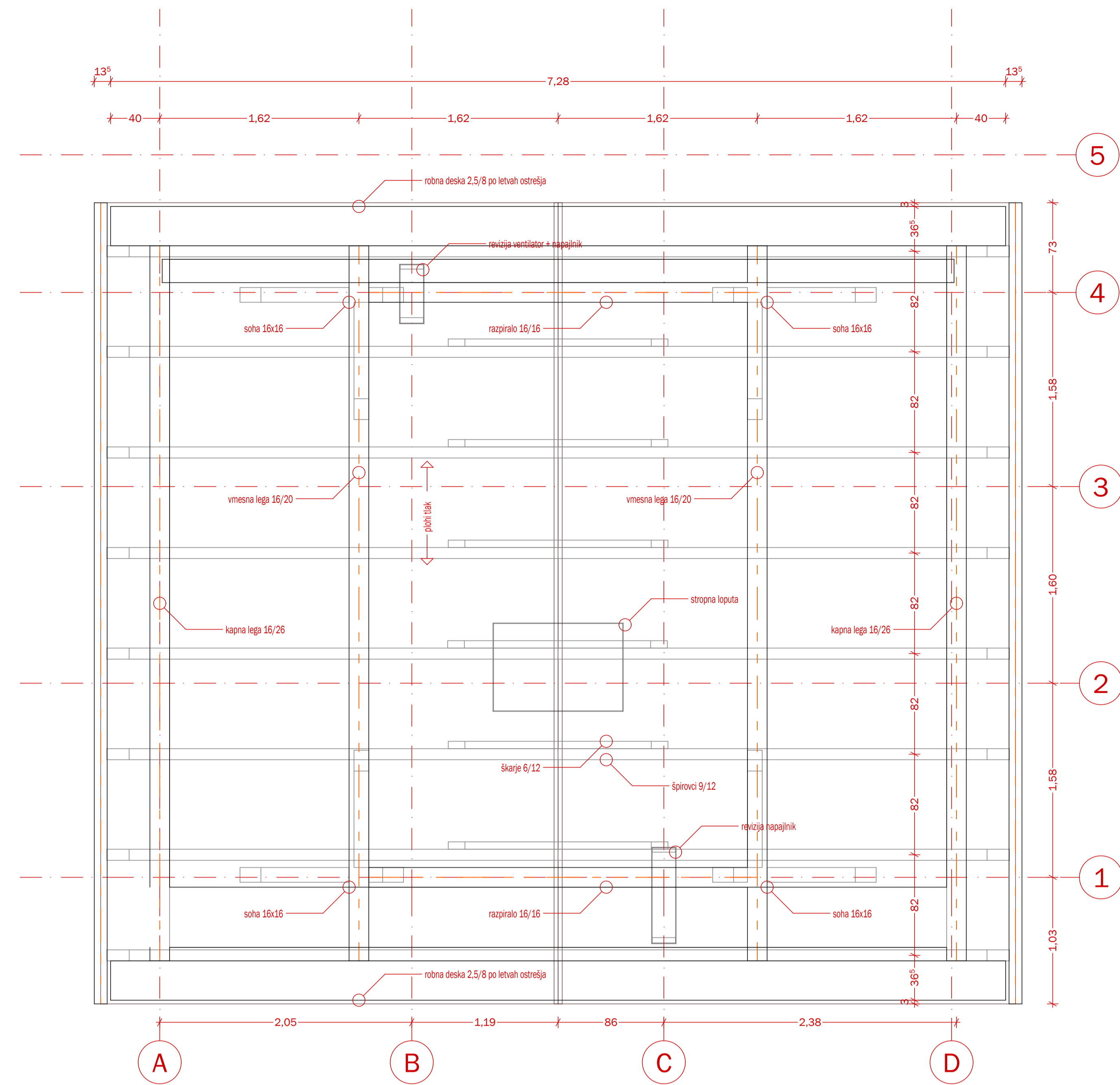
2. ostresje novo 1:25
