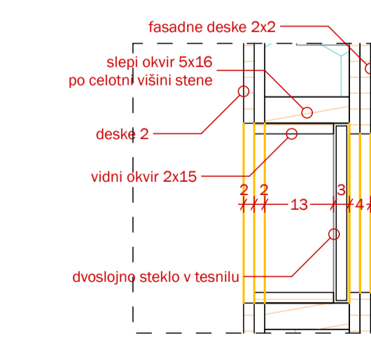
D-T2 1:10
