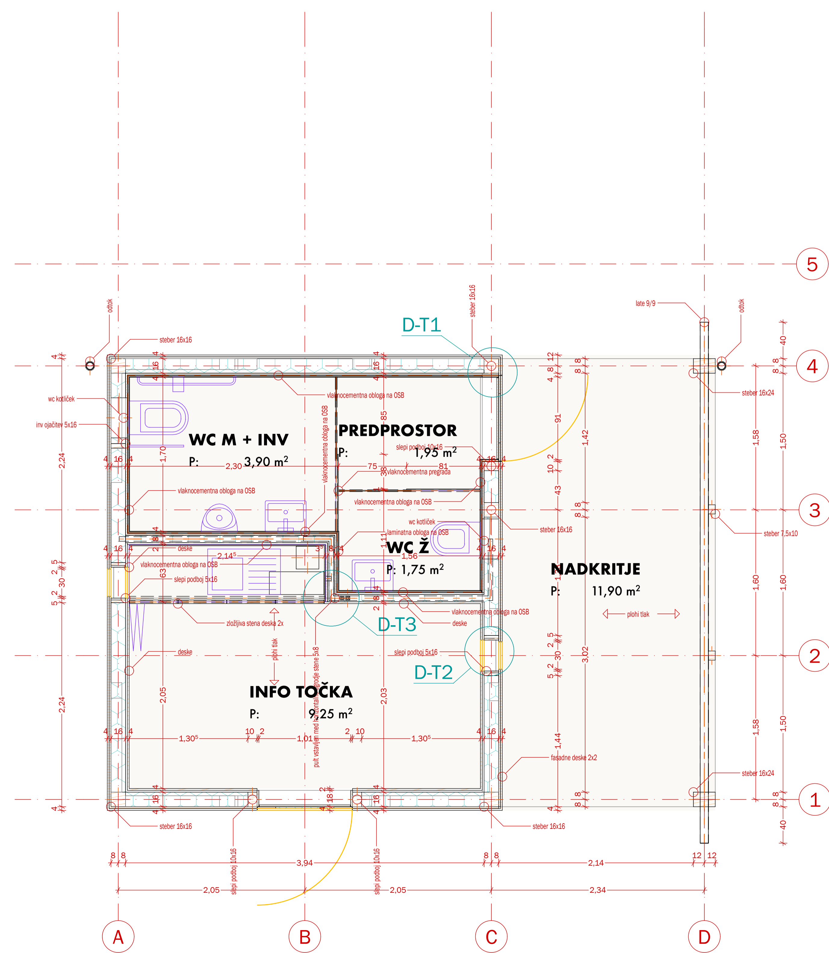
0. tla novo detajli 1:25
