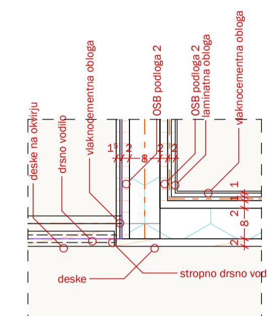
D-T3 1:10
