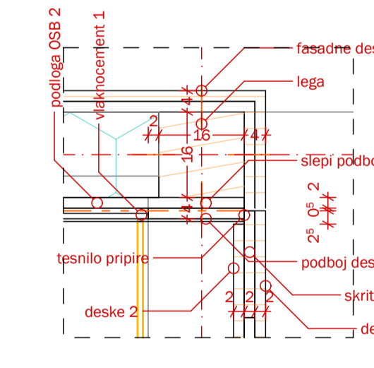
D-T1 1:10
